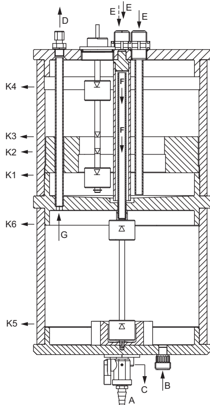
Рис. 4 Реактор и внутренний дозирочный резервуар (OCD-162-5/-10/-30)
