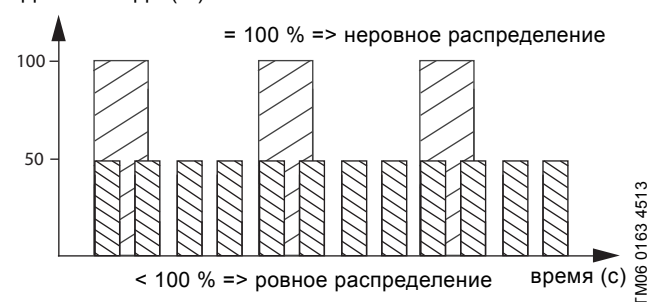
Рис. 35 Распределение объема дозируемого вещества при различной длине хода
