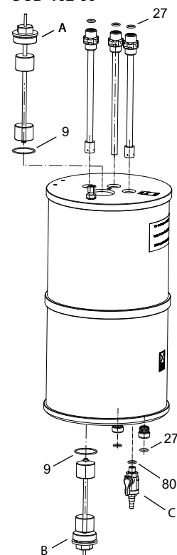
Рис. 44 OCD-162-5, -10, -30: реактор/внутренний дозирующий резервуар
