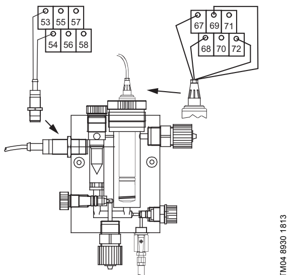
Рис. 20 Схема соединения AQC-D6
