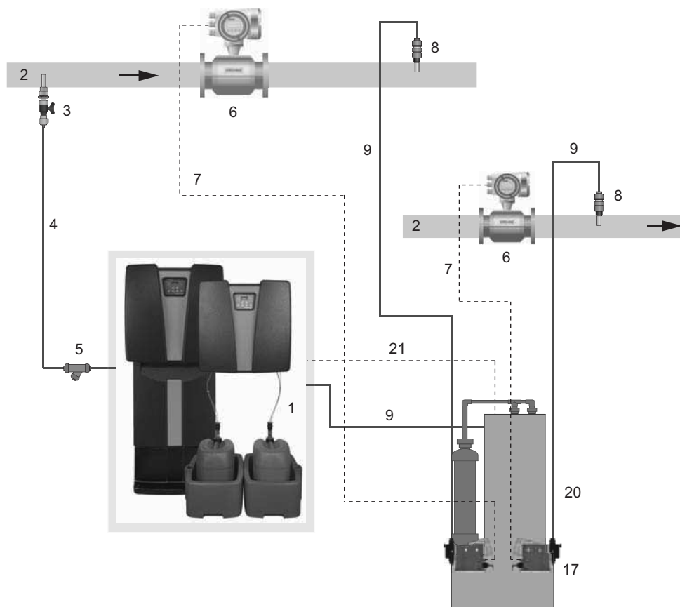
Рис. 13 OCD-162 с внешним дозировочным резервуаром и двумя дозировочными насосами
