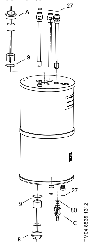
44-сур. OCD-162-5, -10, -30: реактор/ішкі мөлшерлеу сұйықтығы
