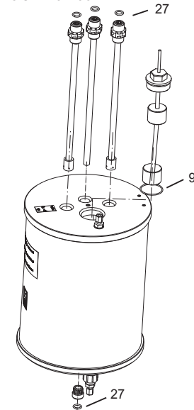
Рис. 45 OCD 162-60: реактор
