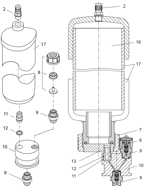
48-сур. OCD-162-30, -60
