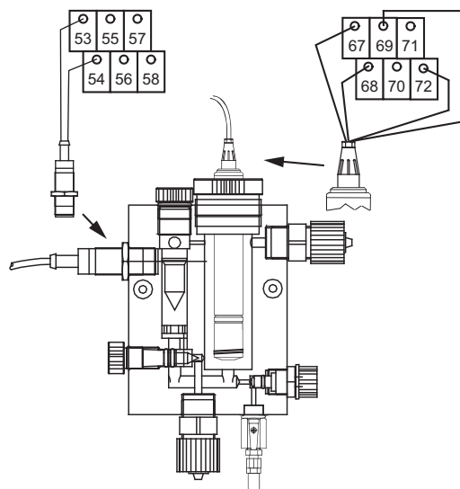
20-сур. AQC-D6 жалғанымының сызбасы
