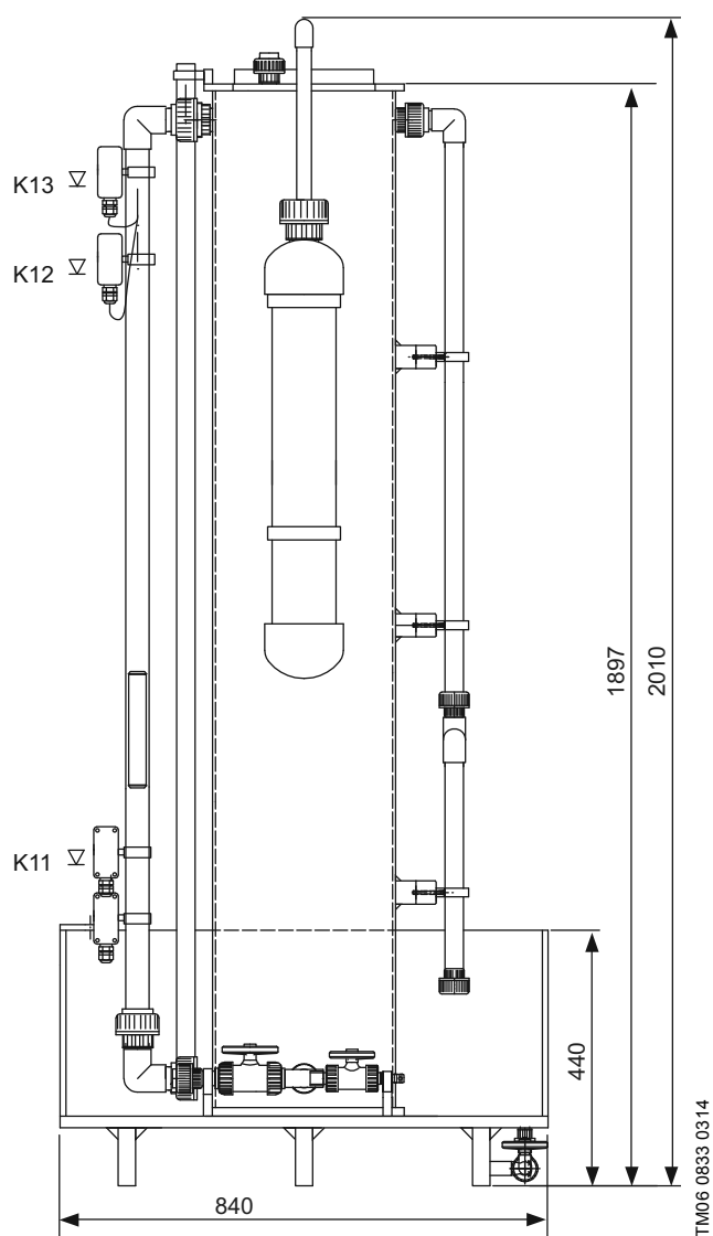
Рис. 50 Внешний дозировочный резервуар
