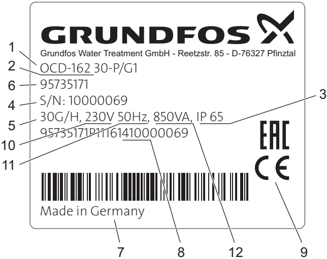
Рис. 7 Фирменная табличка
