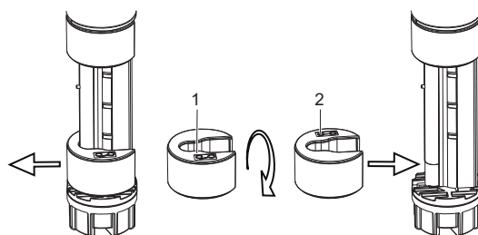
Рис. 14 Изменение полярности поплавка
