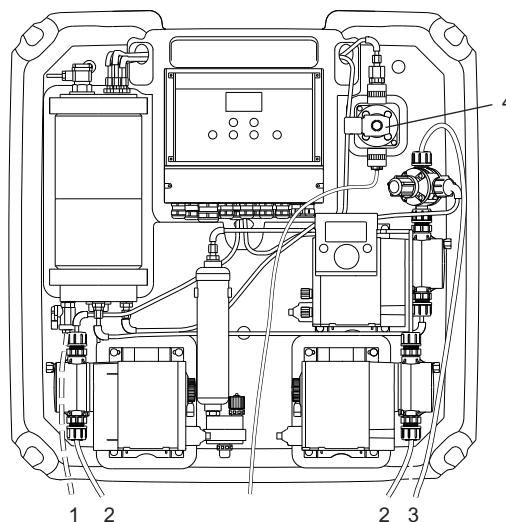
Рис. 15 OCD-162-05 (-10)
