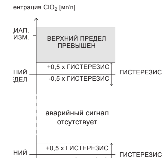
Рис. 34 Пределы концентрации \text{ClO}_2 для аварийного сигнала
